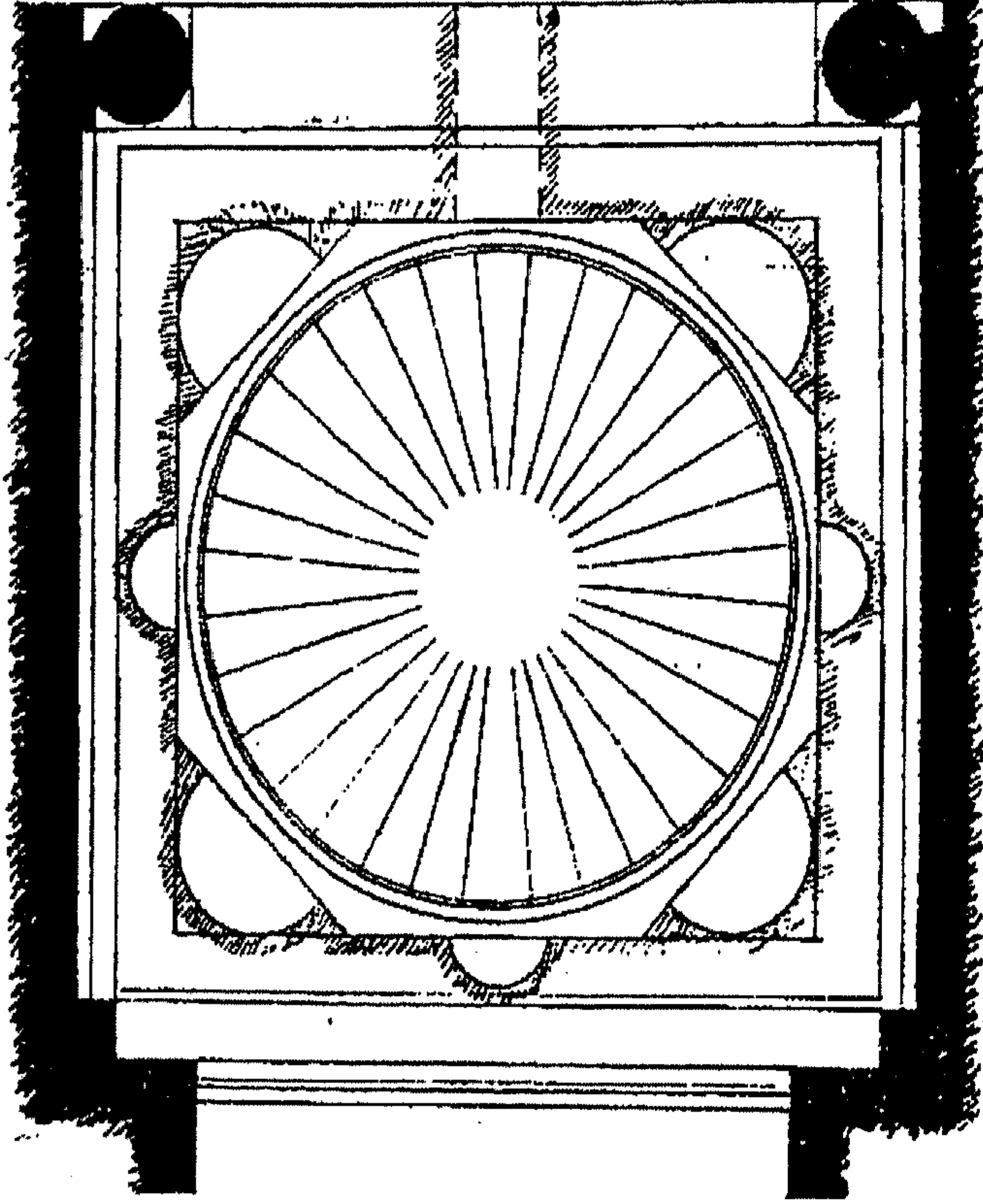
(شكل رقم ١٨) رسم تحليلي لقبة المحراب بجامع القيروان عن د/ أحمد فكري .
